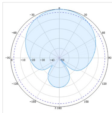
Horizontal (866MHz)
